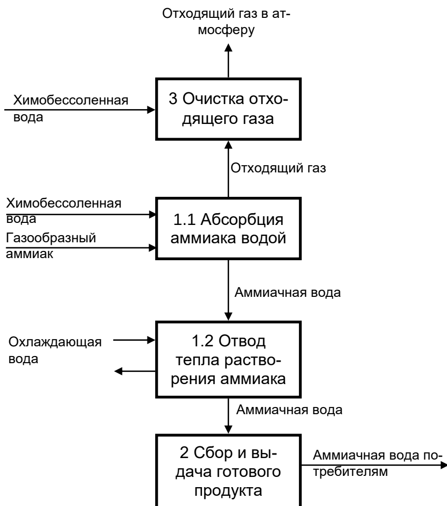
Рисунок 7.8 – Схема технологического процесса
