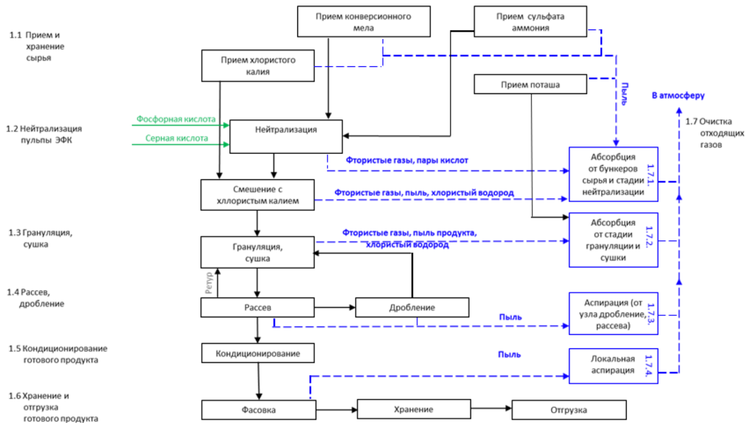
Рисунок 6.5 – Производство PKS / NPKS-удобрений
