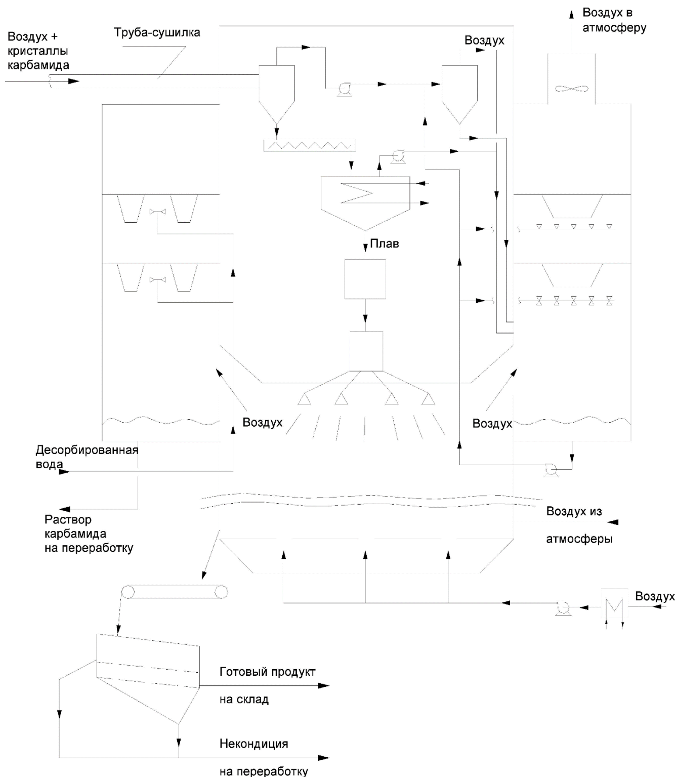
Рисунок 8.18 – Схема узла приллирования фирмы ТЕС
