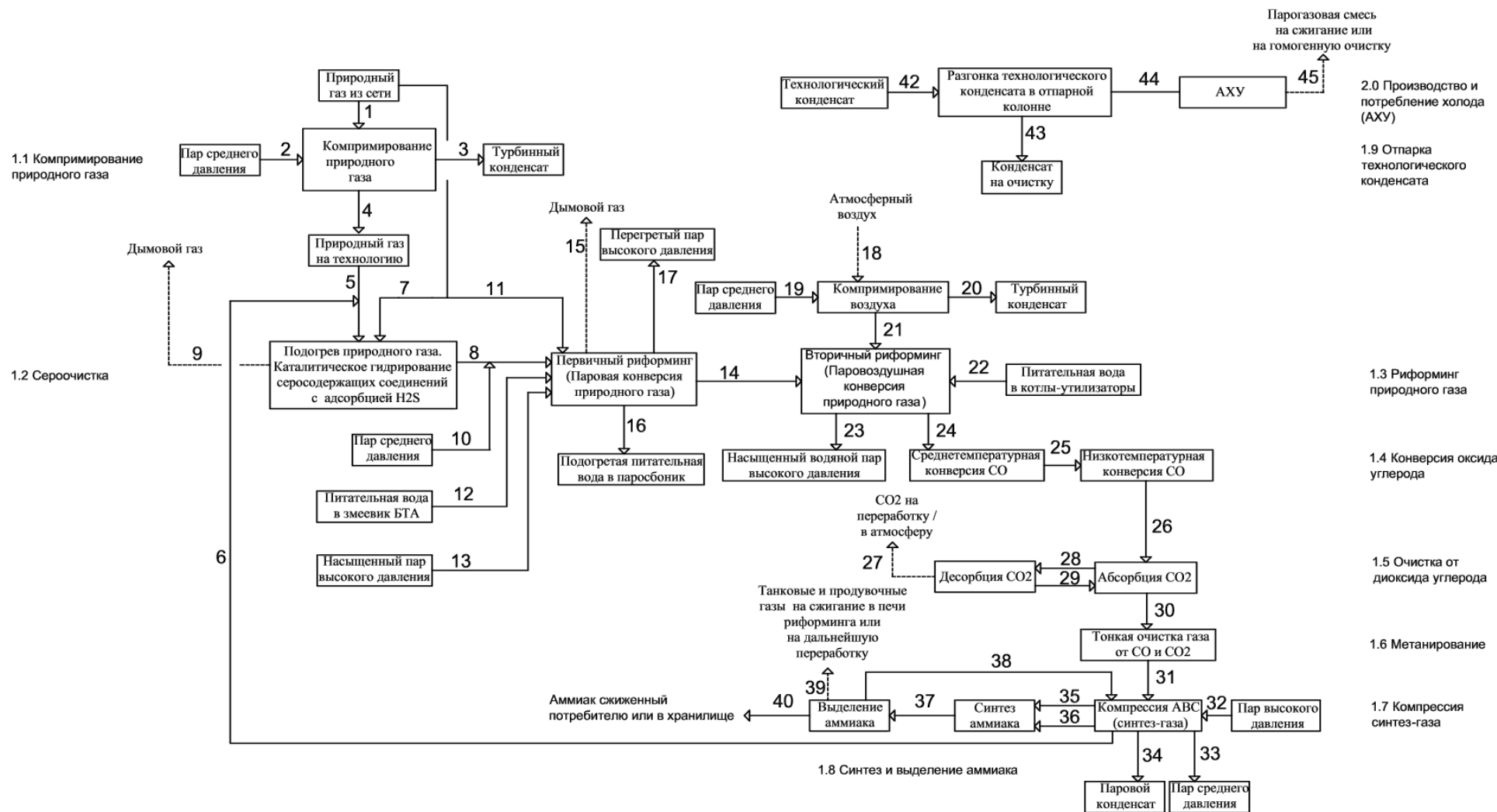
Рисунок 2.2 – Блок-схема технологического процесса производства аммиака
