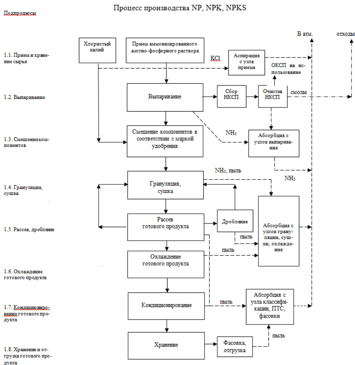
Рисунок 6.8 – Получение NP / NPK / NPKS-удобрений
