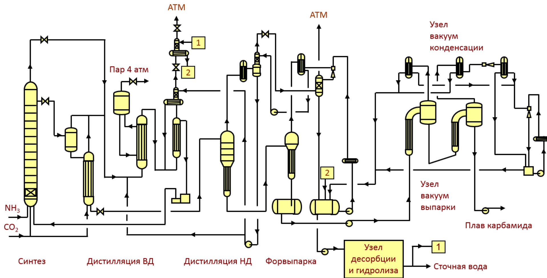
Рисунок 8.379 – Принципиальная схема получения плав карбамида по новой отечественной технологии
