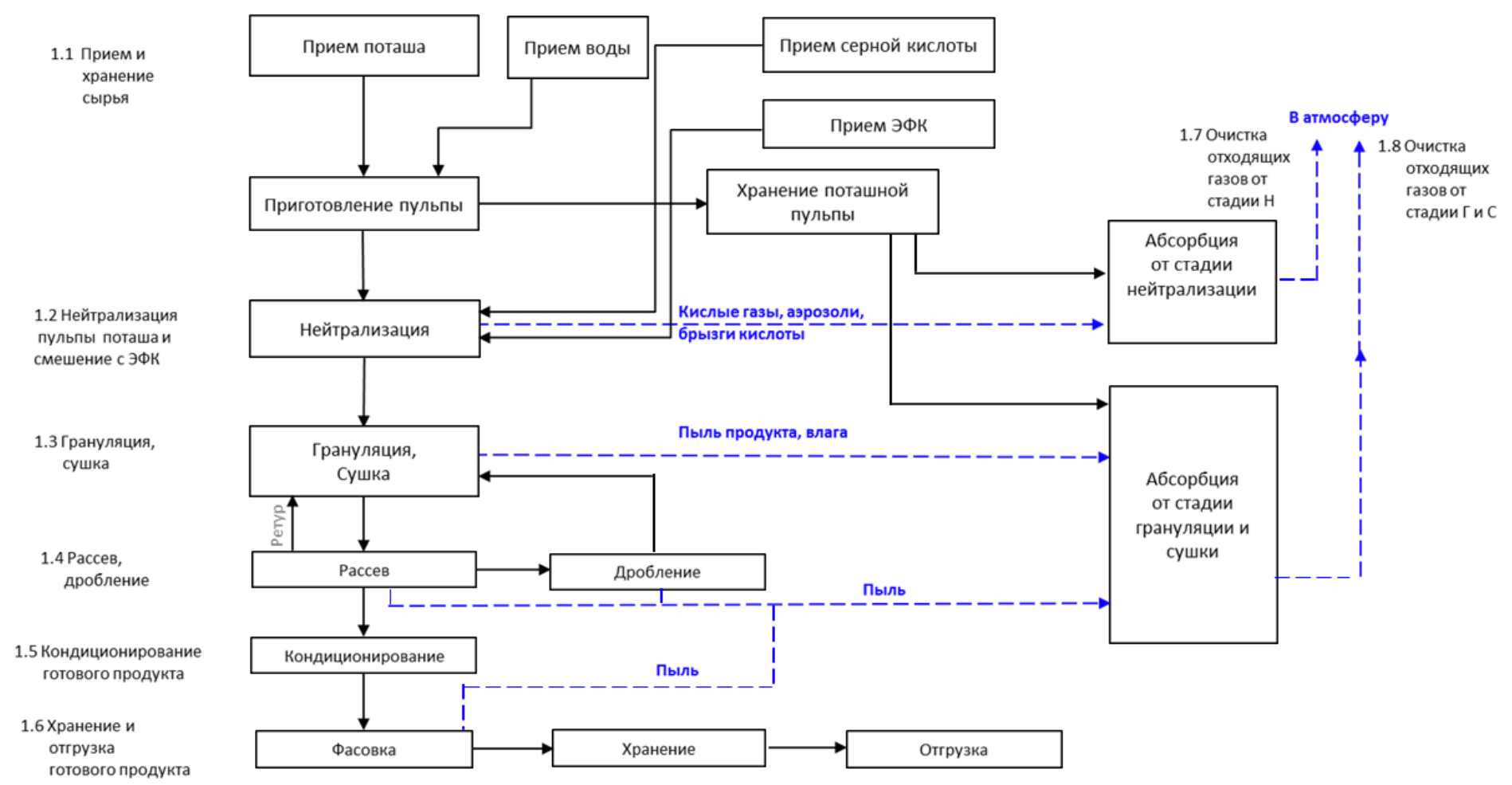
Рисунок 6.1713 – Производство сульфата калия
