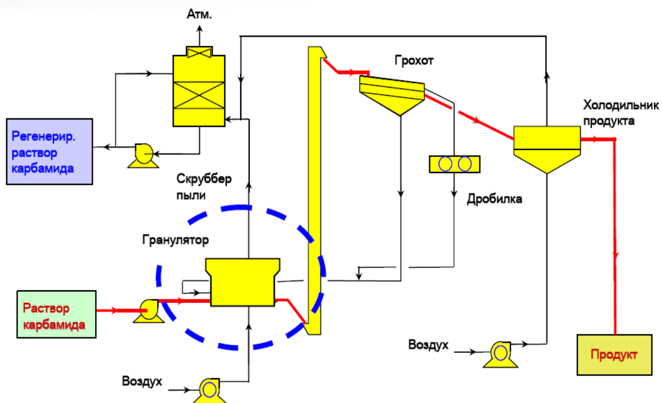
Рисунок 8.20 – Принципиальная технологическая схема процесса грануляции ТЕС
