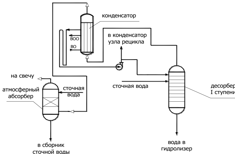
Рисунок 8.34 – Схема установки затопленного конденсатора газов десорбции
